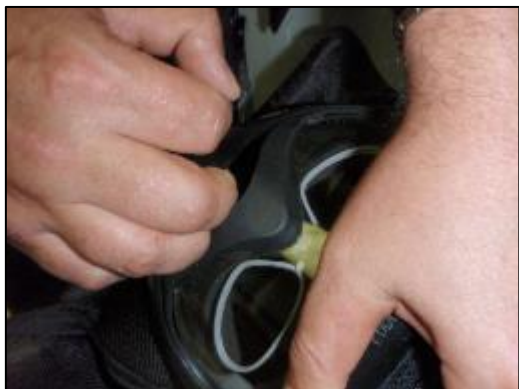
Fig. 10 – Section du nez de la coquille en plastique du Casque Protecteur FX®
